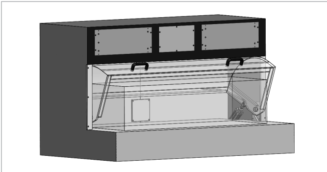
Prüfhaube HB 7000A mit Doppelbreite und Gerätefach 2 x 19" / 5 HE
